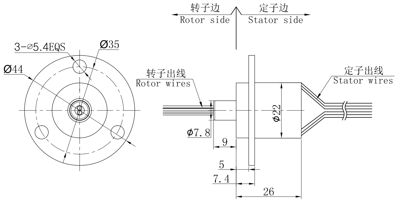
MW1210 外形尺寸图(2环,每环10A)
