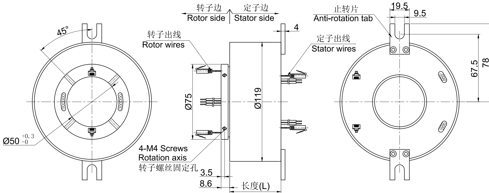
ME2502 size
